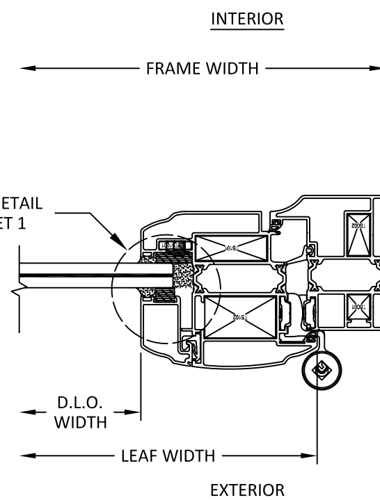
E HORIZONTAL SECTION 5 HINGE JAMB
